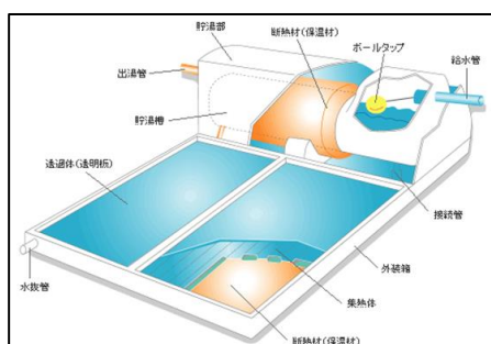
自然循環型
