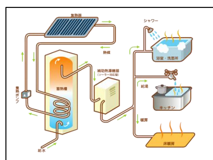
強制循環型
