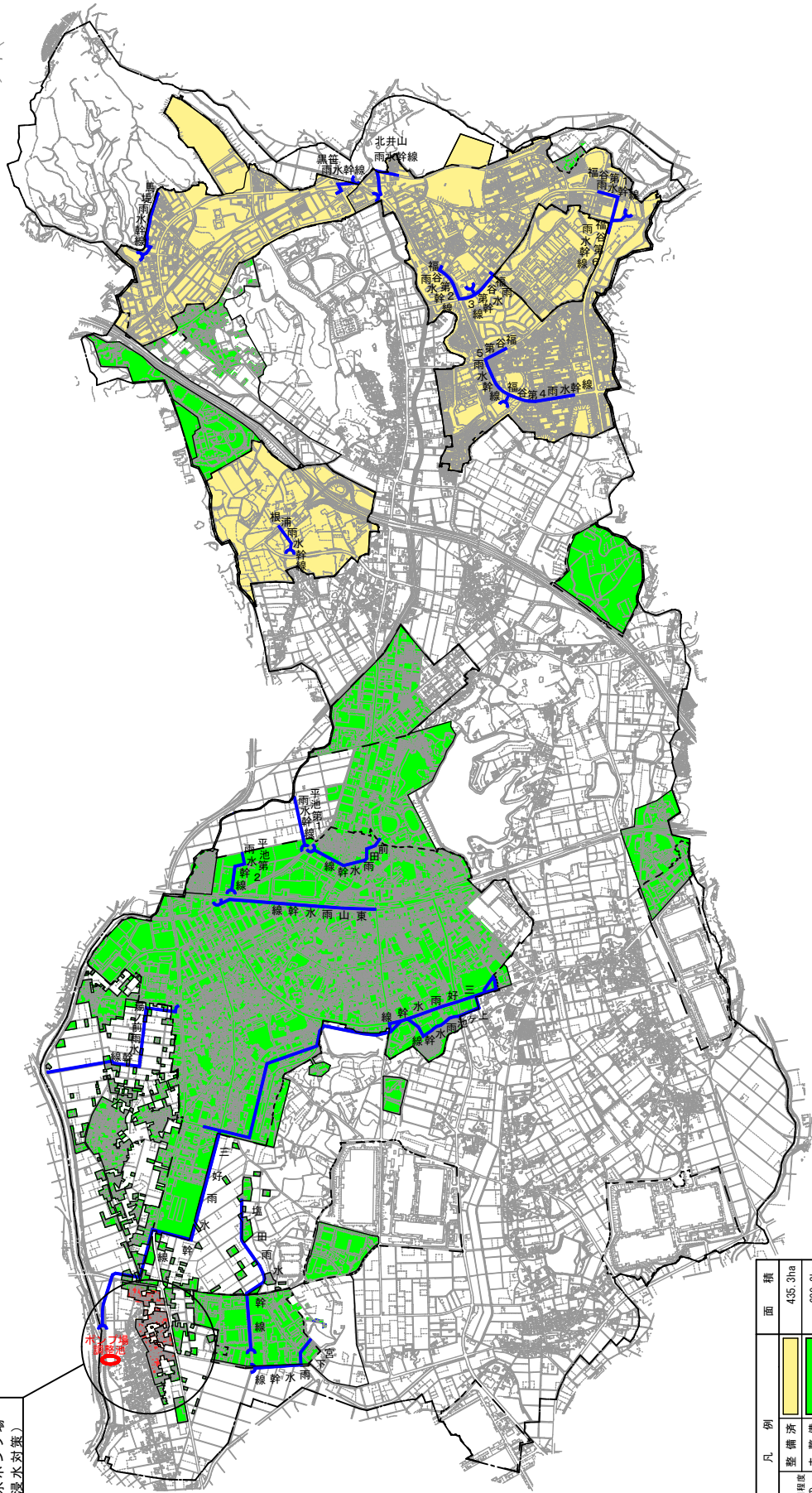
みよし市公共下水道（雨水）施設図
