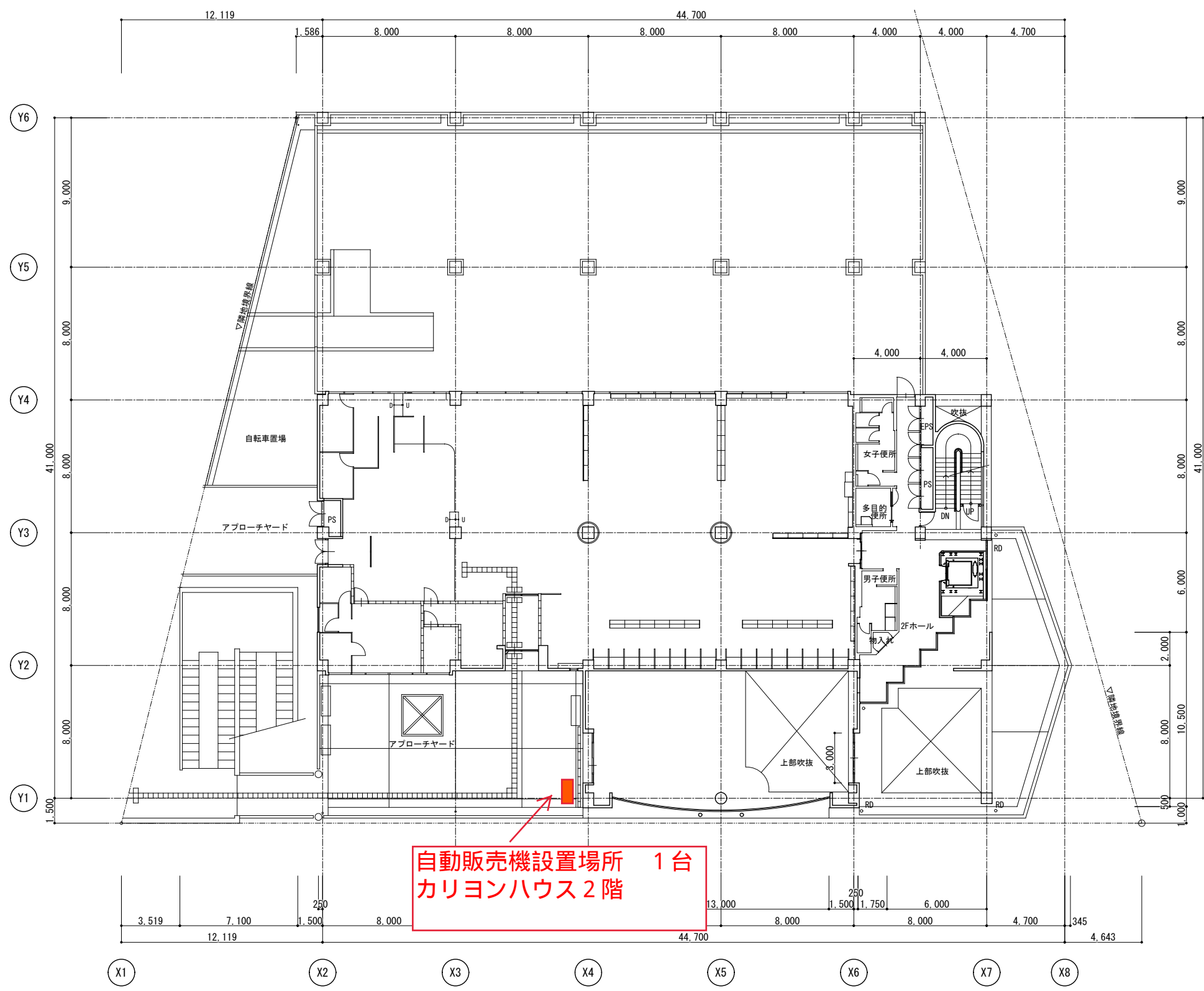
改修後 2階平面図 S=1/200
