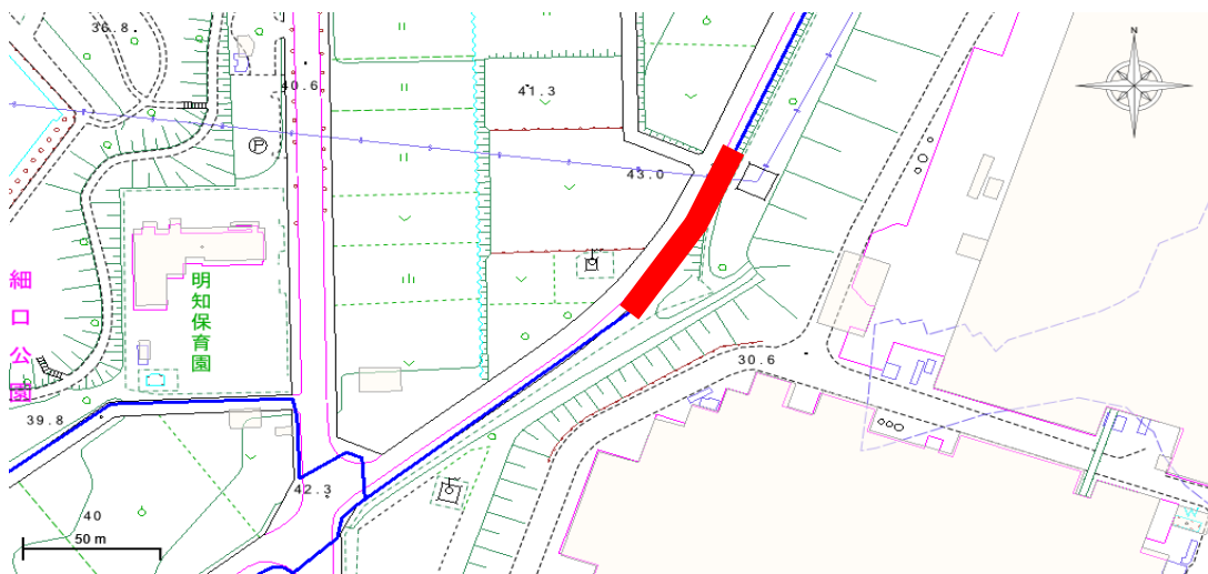
通学路防護柵設置工事[市道下明知打越線]
